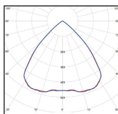
Křivky svítivosti B30-C
